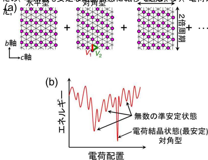
図 2:(a)本物質で起こりうる様々な電荷配置。徐冷すると対角型の電荷配置をとるが、急冷すると様々な電荷配置が混ざり合ったガラス状態になる。 V_1 と V_2 は二等辺三角格子上的クーロン斥力を表している( V_1 > V_2 )。(b)様々な電荷配置に対するエネルギー状態。水平型が最も安定な電荷配置となるが、急冷により準安定状態に落ち込むとガラス状態になる。
