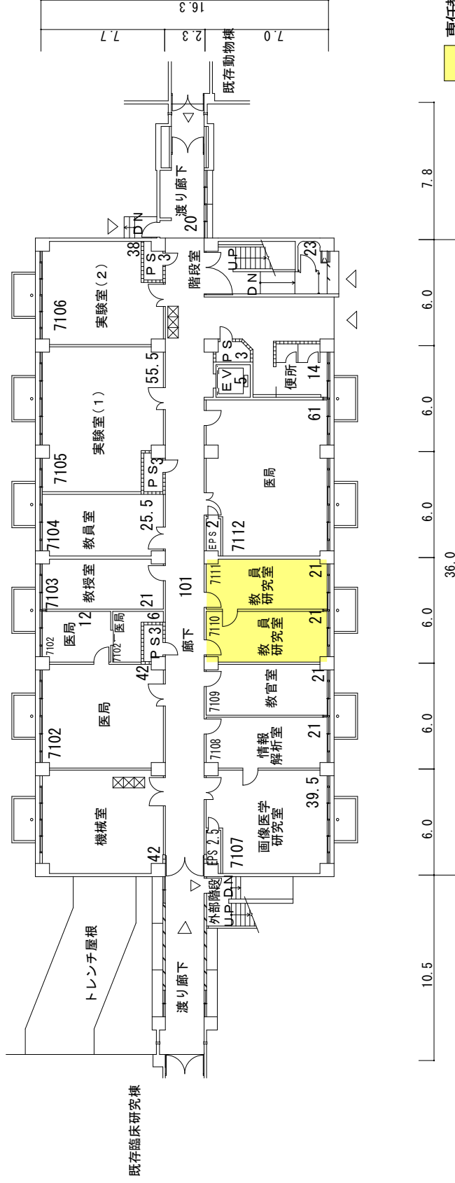
024 院生研究棟 1階平面図 S=1/300
